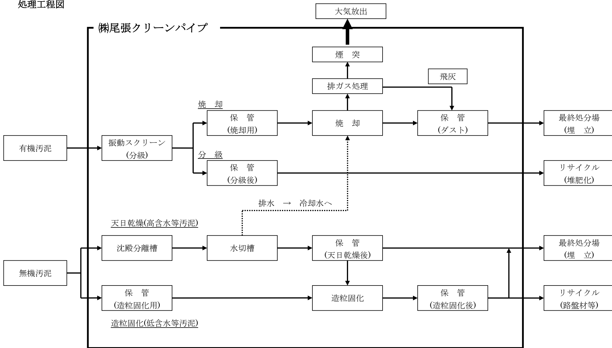
処理工程図
